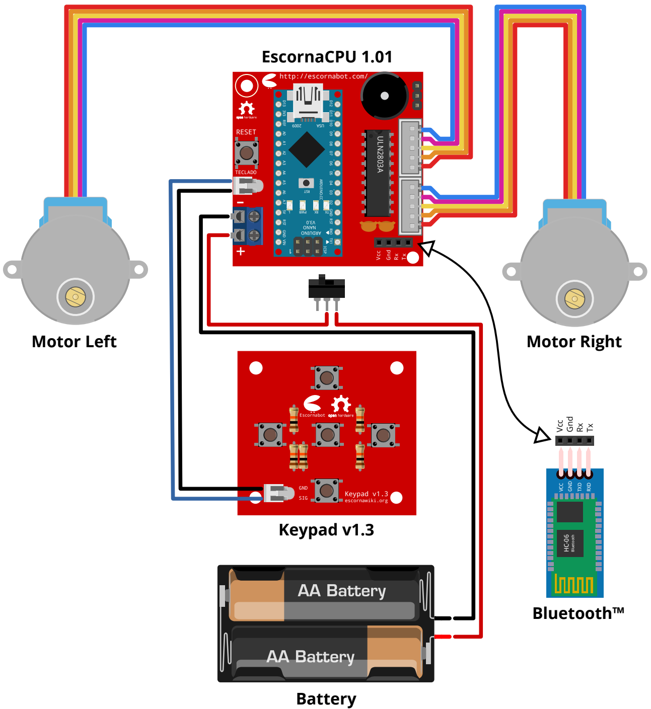
Esquema de conexión de un Escornabot «Brivoi»
